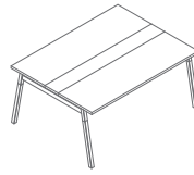
SW26 1600 / 1210 / 740 59.7 kg
