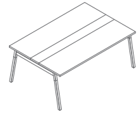
SW28 1800 / 1210 / 740 67.3 kg
