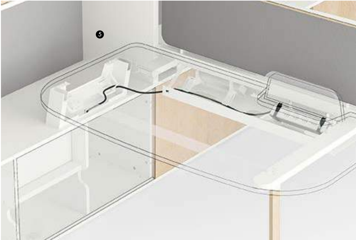
5 IT Cablaggio EN Wiring FR Câblage DE Verkabelung ES Cablaje RU Проводка
